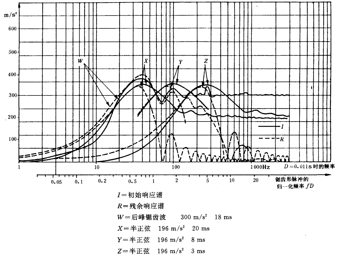
图 B8 300\text{ m/s}^2 18 ms 的后峰锯齿波的冲击谱与 200\text{ m/s}^2 及持续时间为 3 ms 和 20 ms 之间的半正弦脉冲的冲击谱的比较
